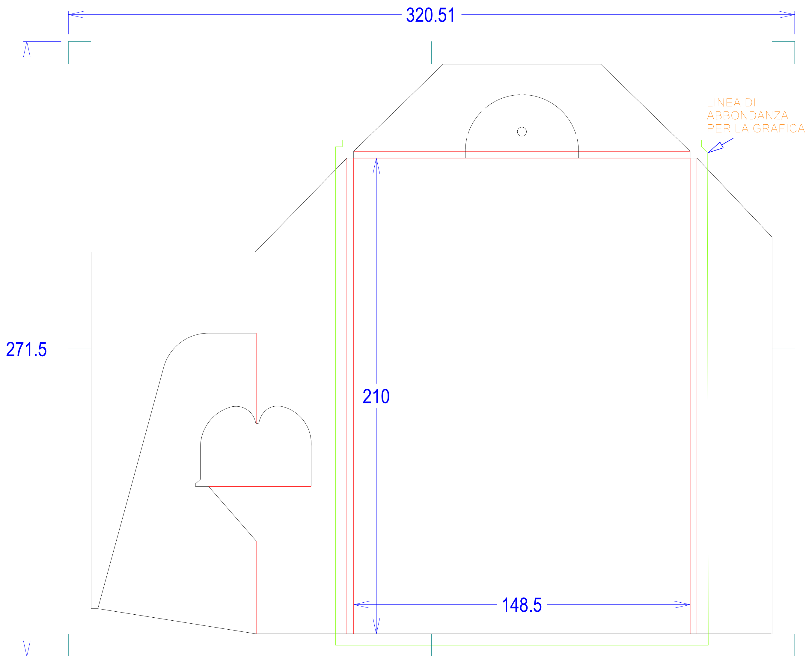
PINZA LATO STAMPA COD. 800_3003-11_DIS1
